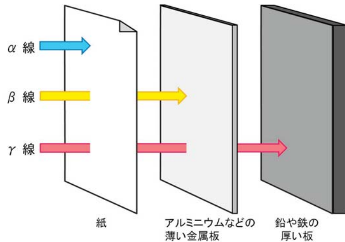
図 1.6 \alpha 線、 \beta 線、 \gamma 線の透過力
