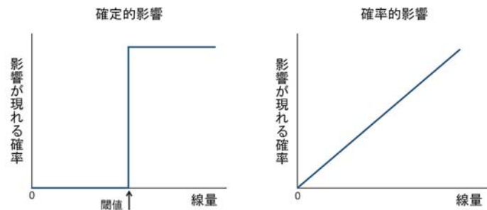
図 2.1 浴びた放射線の量と、障害が現われる確率とのおよその関係。
