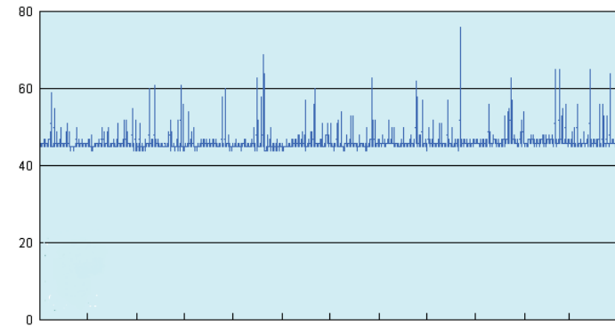
図1.5 茨城県水戸市での、空間放射線量率の日ごとの変化。縦軸の単位は、ナノ・グレイ/時。ウェブサイト「日本の環境放射能と放射線」掲載のものを一部改変。
